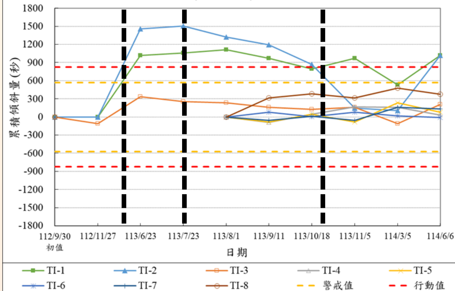
傾度盤(TI 垂直向)歷時曲線圖
